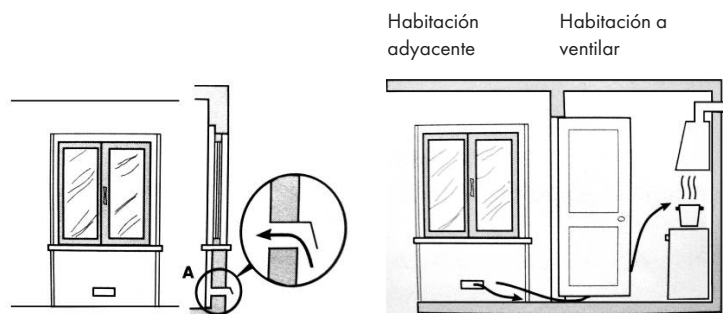
Ejemplo de aberturas de suministro de aire para el aire de combustión
