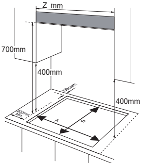
Benötigte Abstände bei der Montage mit Dunstabzugshaube
