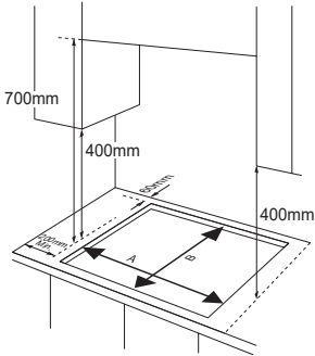
Benötigte Abstände bei der Montage ohne Dunstabzugshaube
