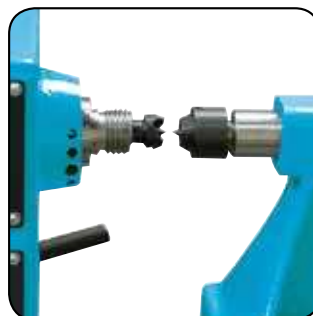
Broche d'entraînement CM2 filetée M33 x 3,5 Aandrijfspil CM2 met schroefdraad M33 x 3,5
