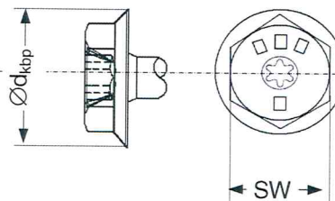
Sechskantkopf mit Bund
