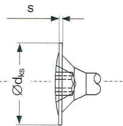
Linsenkopf mit Scheibe
