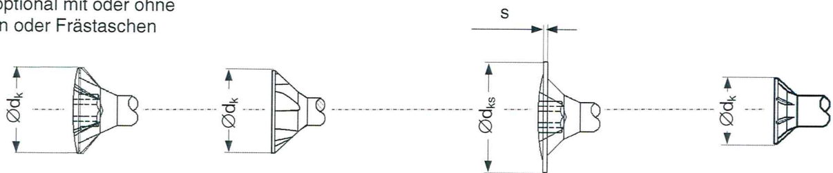
Linsenkopf Reibminderungstaschen/F6 Linsenkopf mit Scheibe Kleiner Kopf
