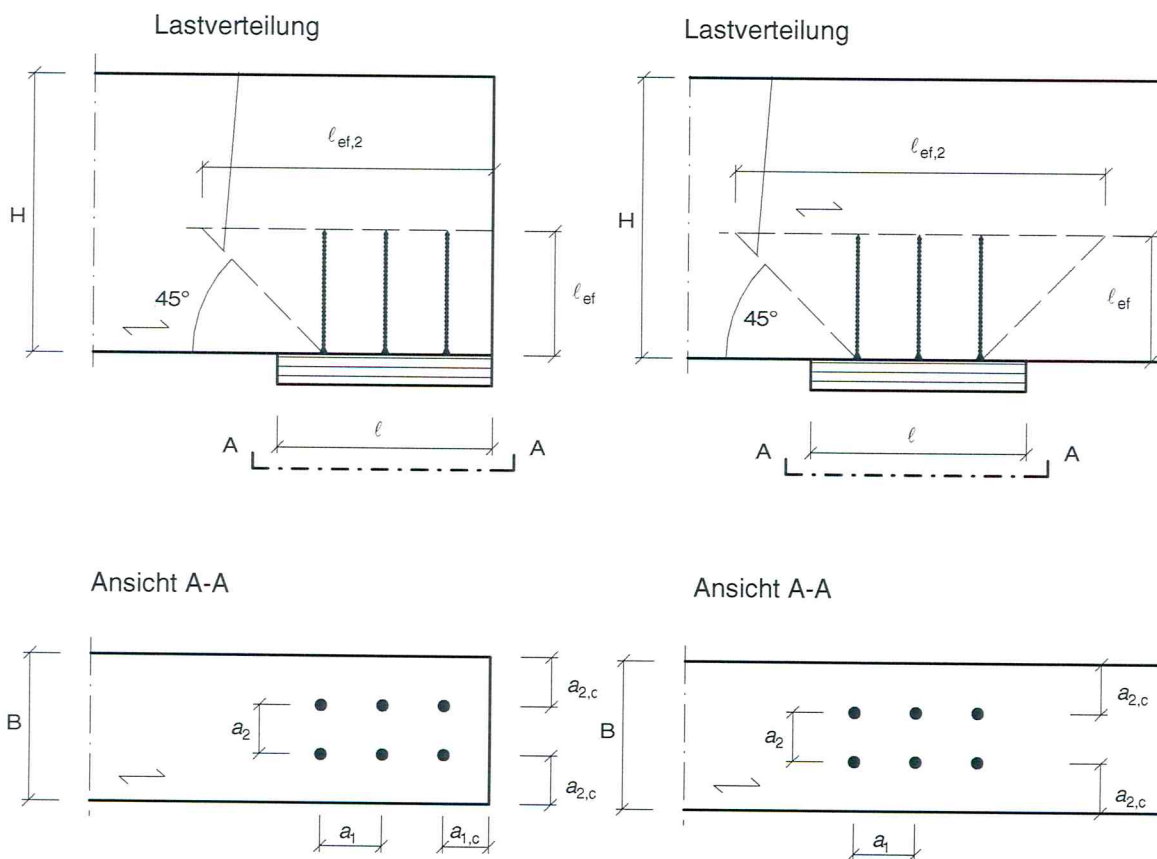
Abbildung 2.1: Verstärktes Endauflager (links) und verstärktes Zwischenaflager (rechts)
