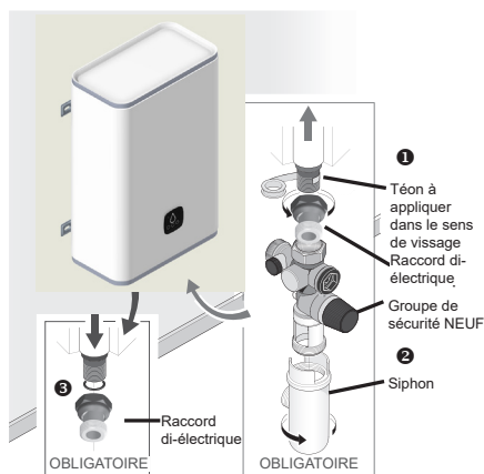
Branchement eau froide
