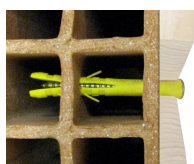
Cheville CQLV - vue en coupe dans la brique
