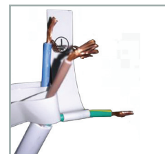
Câble d'alimentation
