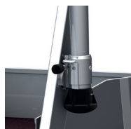
Système de blocage et déblocage du garde-corps de sécurité.
