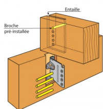
Installation des broches
