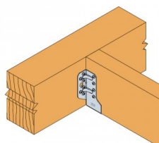
Clouage total sur bois
