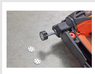
Eurocode 019891 Ensemble porte rondelle PULSA 27P
