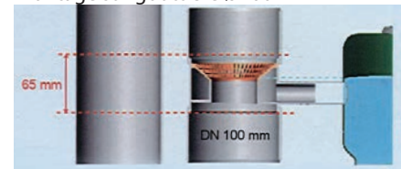
Montage sur gouttière Ø100
