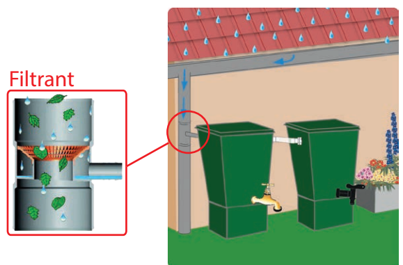
Montage sur gouttière Ø80
