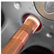
Dégrillage d'écrous de roue
