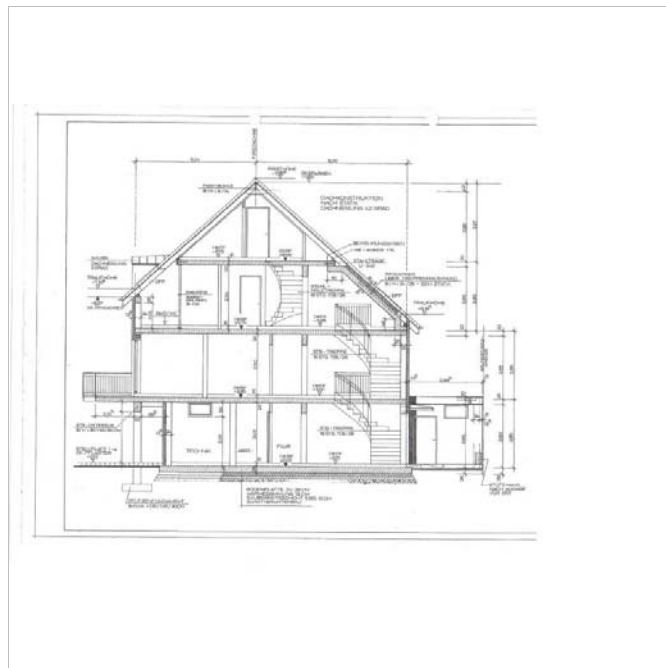
Grund_Querschnitt
