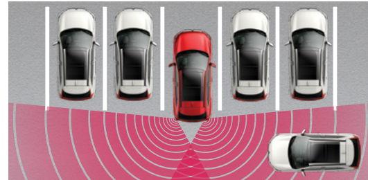
מערכת התרעה על תנועה אחורית חוצה* Rear Cross Traffic Alert - RCTA
