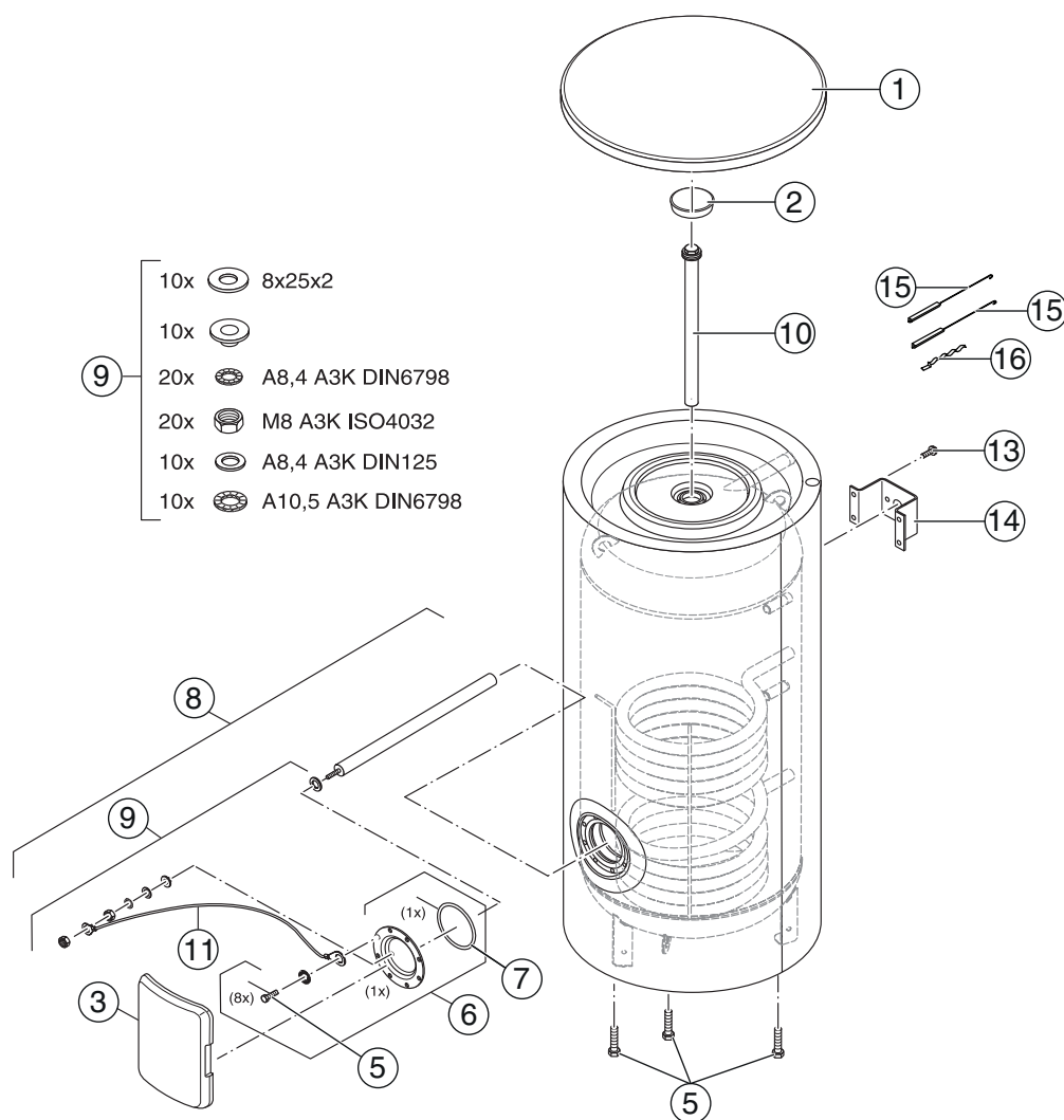
Fig. 25 Pièces de rechange pour SU80/5, SU100/5
