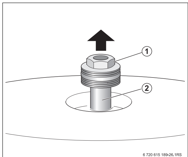
Fig. 20 Contrôler l'anode en magnésium supérieure SU80/5, SU100/5
