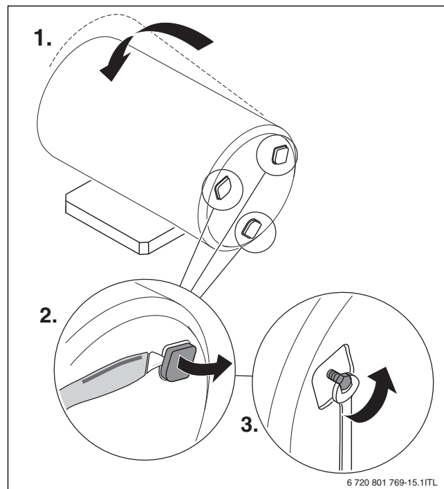
Fig. 8 Colocar el acumulador de agua caliente y descubrir las patas regulables.
