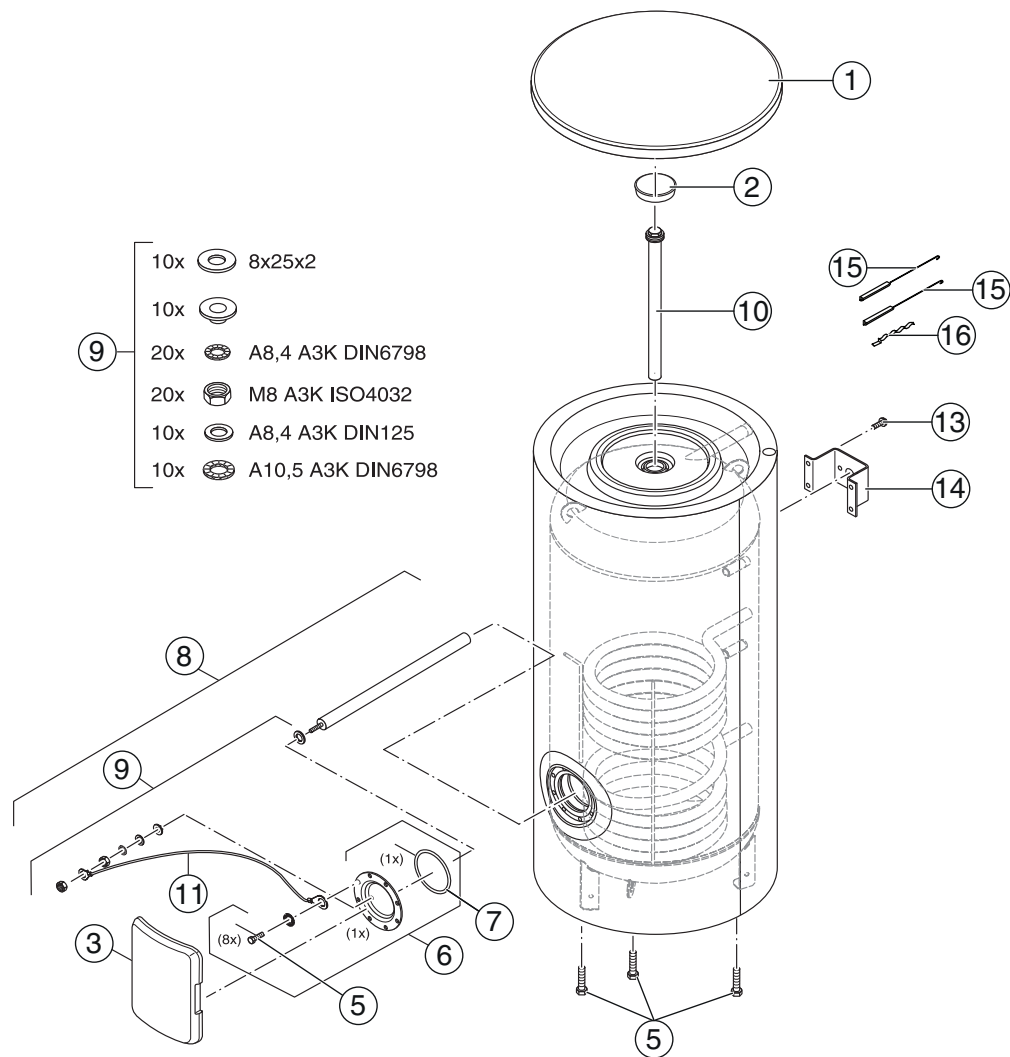
Fig. 25 Piezas de repuesto para SU80/5, SU100/5
