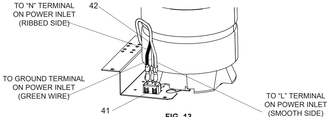
FIG. 13 220V/240V Power Inlet Detail 220V/240V potencia entrada detalle 220V/240V alimentation détail
