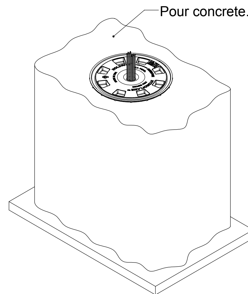
POUR CONCRETE. (Fig. 5)
