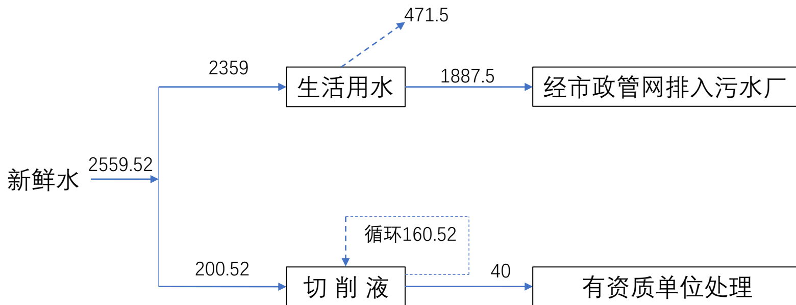
水平衡图 单位m 3 /a
