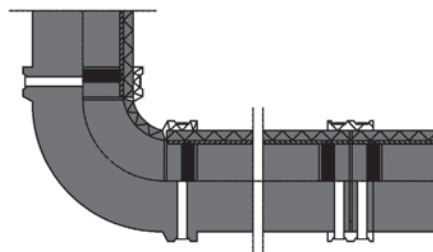
Valmiiksi eristettyjen kanavien ja kanavaosien liittäminen toisiinsa.
