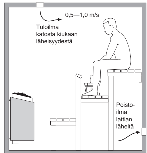
Löylyhuoneen ilmanvaihto
