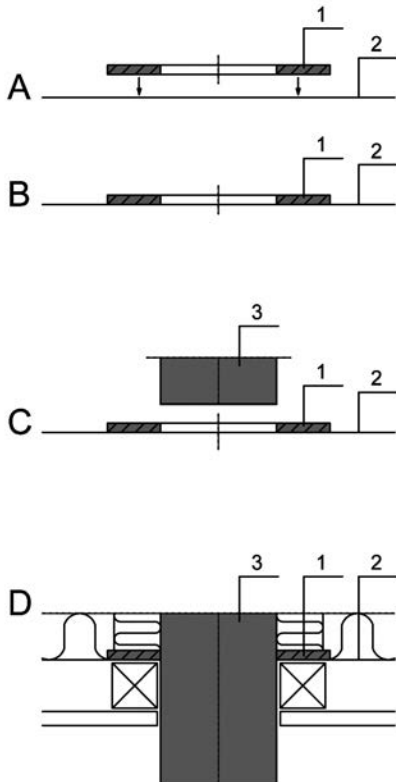
1 = Tiivistyslaippa 2 = Höyrösulku 3 = Eristämätön kanava
