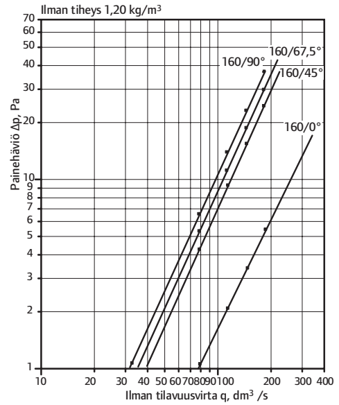
Joustava kanavaosa 160x0-90°
