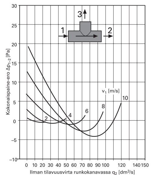
T-kappale 125/125
