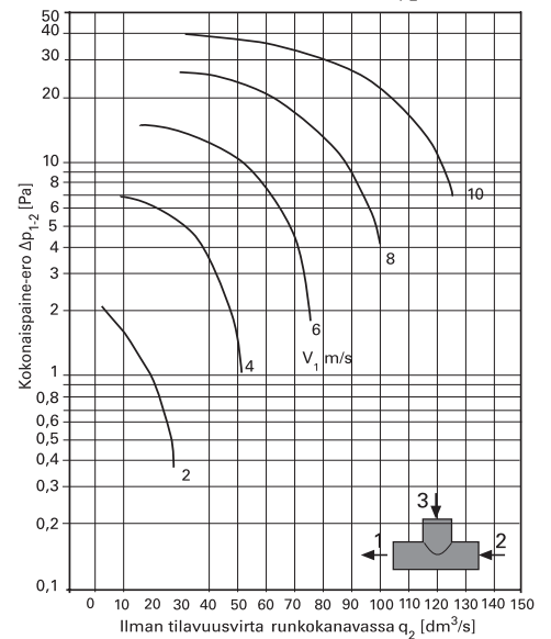
T-kappale 125/125
