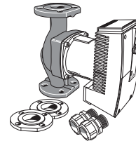
Ulkoinen lämmön- keruupumppu (vain 40 ja 60 kW)
