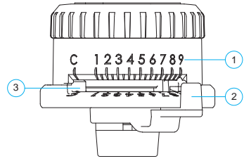
Kuva 10. Esisäättöarvon asettaminen
