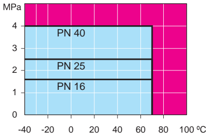
Kuvaaja 4. Paine-lämpötilakuvaaja, kaasupalloventtiilit DN 10–50
