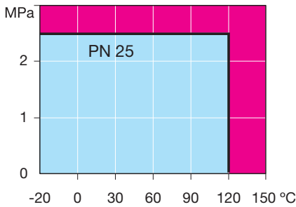
Kuvaaja 1. Paine-lämpötilakuvaaja
