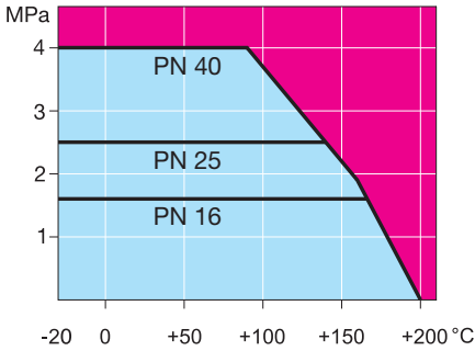
Kuvaaja 3. Paine-lämpötilakuvaaja, teräspalloventtiilit ja haponkestävät teräspalloventtiilit DN 10–50
