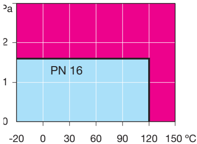
Kuvaaja 2. Paine-lämpötilakuvaaja,
