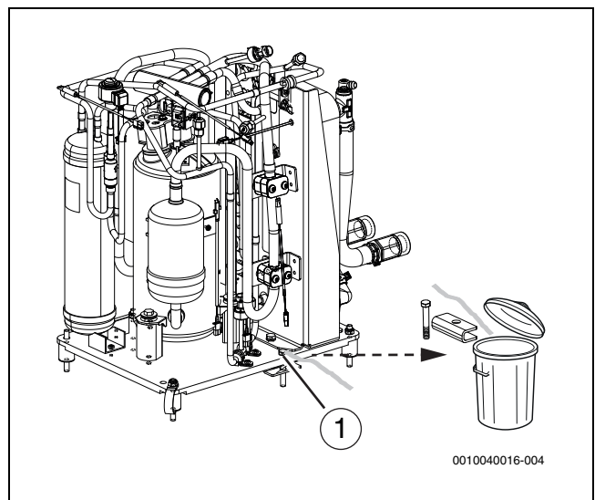
Kuva 32 Kuljetusruuvi
