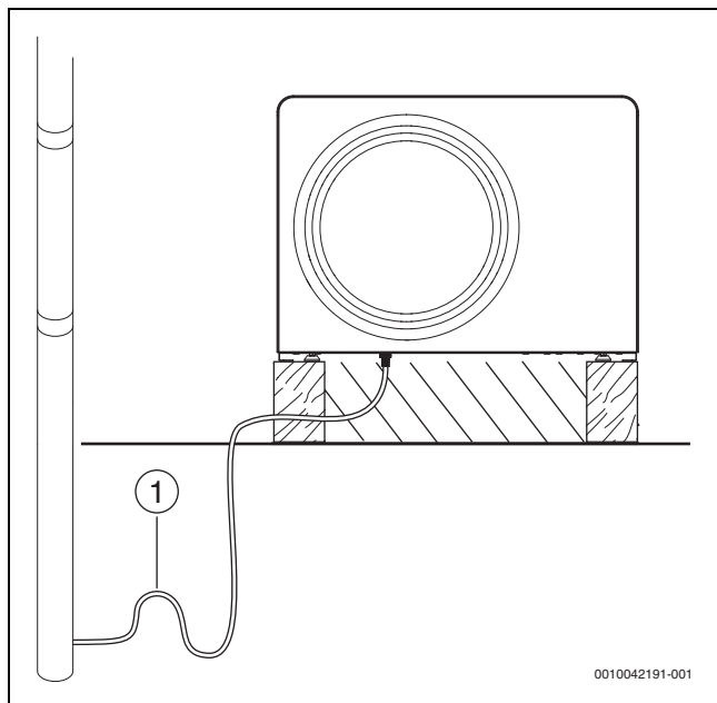
Kuva 26 Kondenssiveden poisto viemäriin/sadevesiviemäriin
