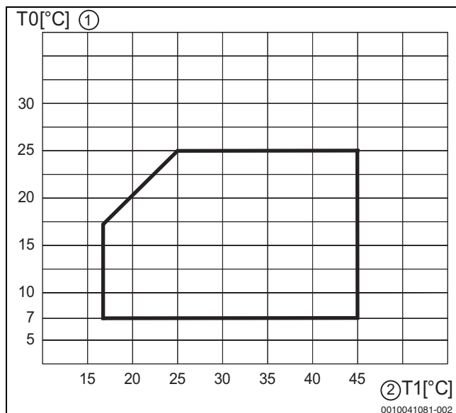
Kuva 44 Lämpöpumppu jäähdytystilassa
