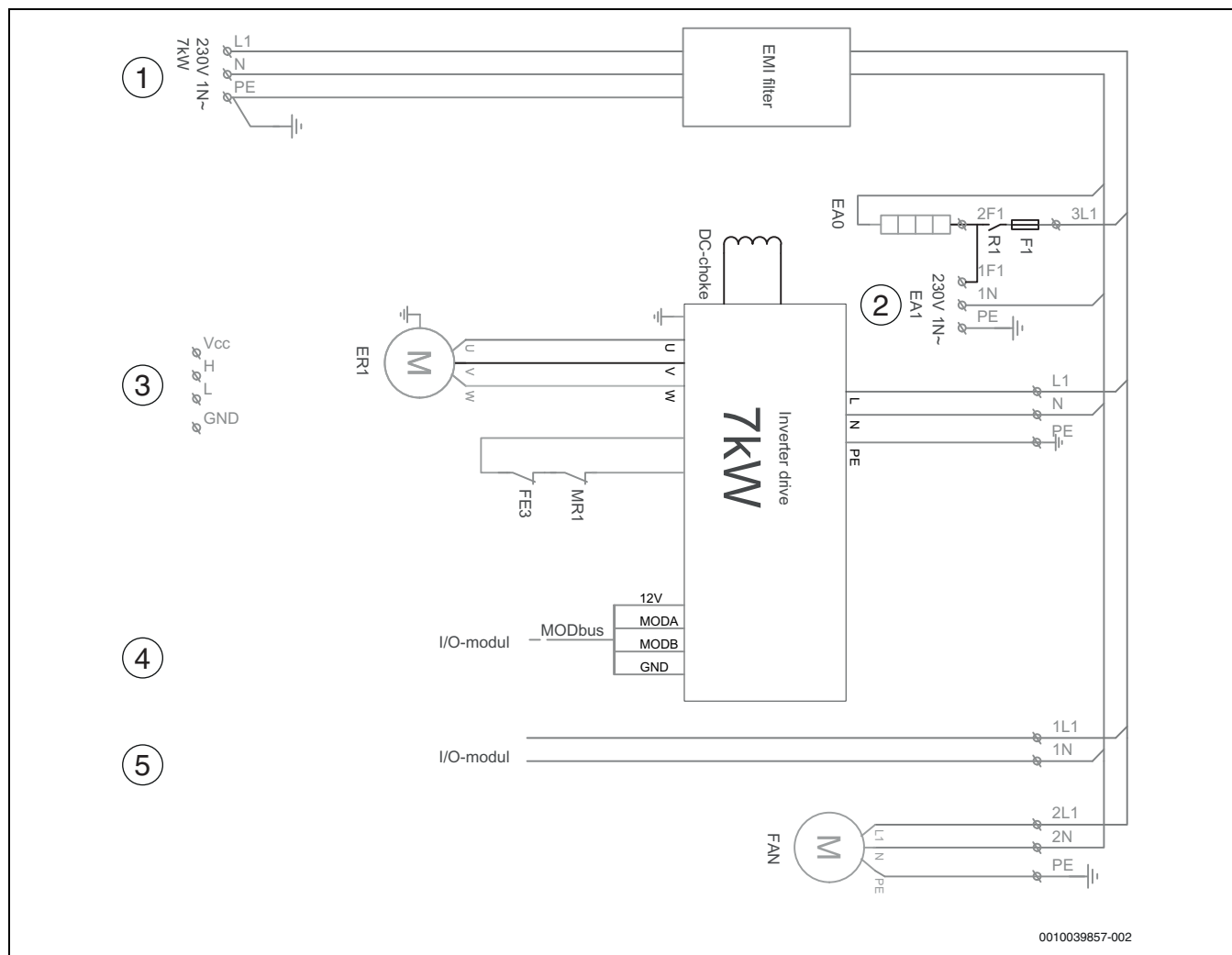
Kuva 46 Invertterin sähköpiirikaavio
