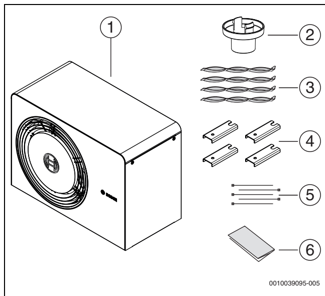
Kuva 1 Vakiotoimitus
