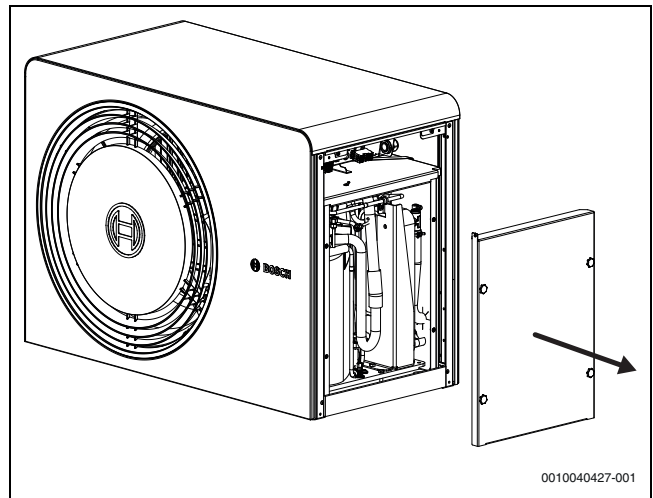
Kuva 31 Kylmäainelaatikon kansi
