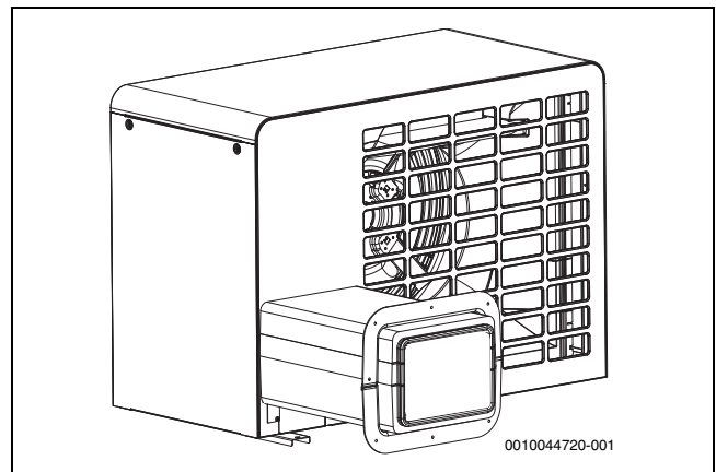
Kuva 22 Asennussarja, seinäkiinnitys
