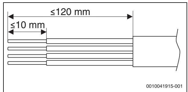
Kuva 34 CAN-väyläjohtojen kuoriminen
