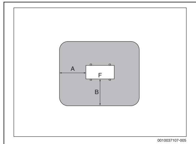
Kuva 9 Maahan tai katolle sijoitetun lämpöpumpun suoja-alue
