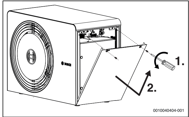
Kuva 30 Sivukansi
