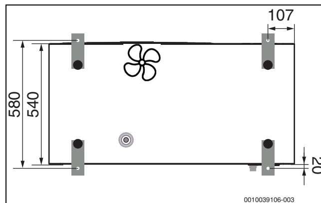
Kuva 5 Lämpöpumpun mitat, ylhäältä
