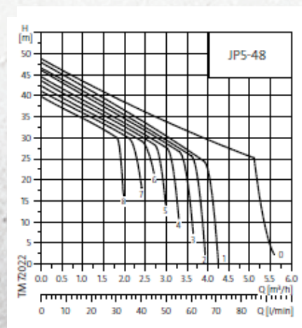
Pumpun tuottokäyrä
