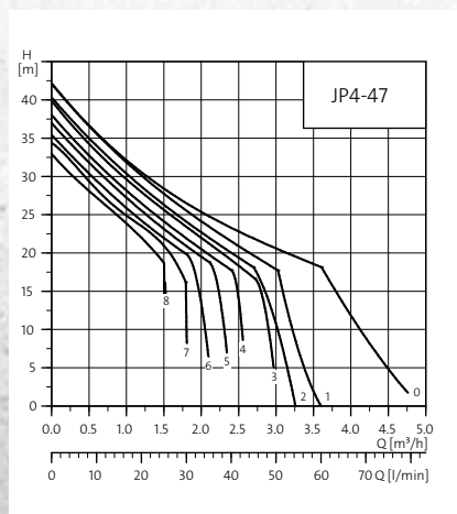
Pumpun tuottokäyrä
