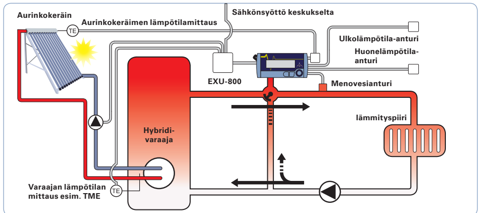
Kuva 4. Periaatekuva hybridilämmityksestä, jossa lämmönsäädin ohjaa aurinkokeräimen ja varaajan välistä latauspumpppua sekä toimii lämmitysjärjestelmän säätimenä ulkolämpötilan ja menoveden lämpötilan perusteella.
