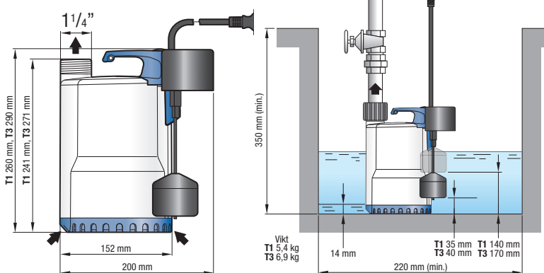
Måttbild RIVER Drain T1 GE och T3 GE
