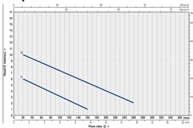
Pumpkurvor RIVER Drain T1 GE och T3 GE
