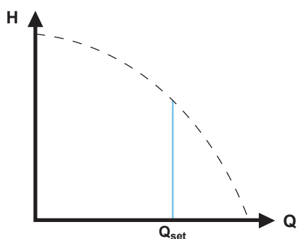
Vakiovirtaaman käyrä
