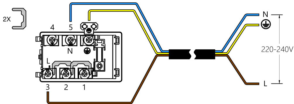
YKSIVAIHEKYTKENTÄ 220-240 VAC :
