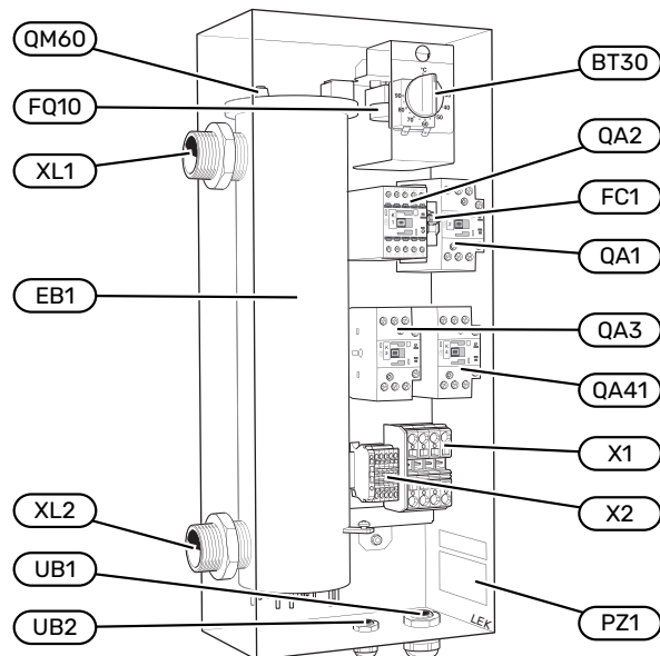
Komponenttiluettelo
