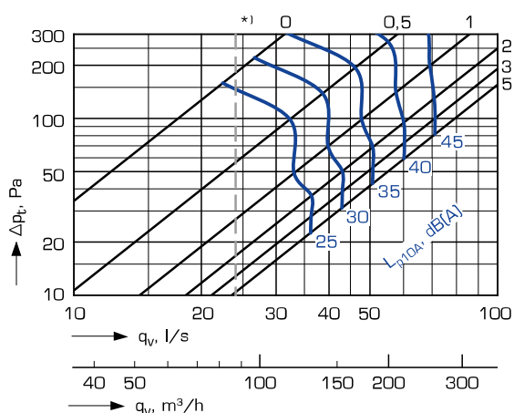
DY(C,K)H-160-4 + ATTS-125-160-1 - rako 0 mm
