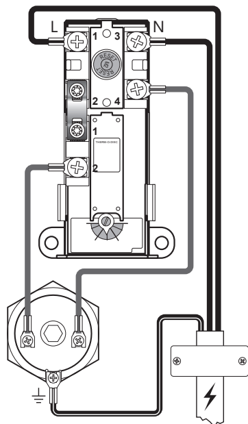
Kytkeäntärsiö - 3 kW - 1x230V Yläsäiliön normaalikytkentä
