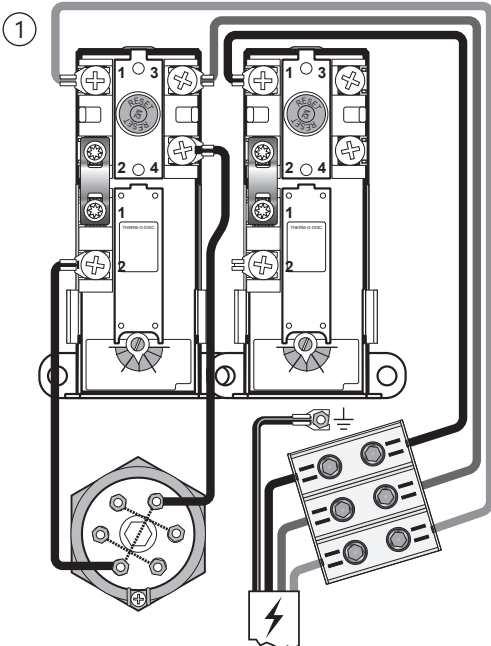
KytKentäkaavio - 3 kW - 3x230V Alasäiliön vaihtoehtoinen kytKentä
