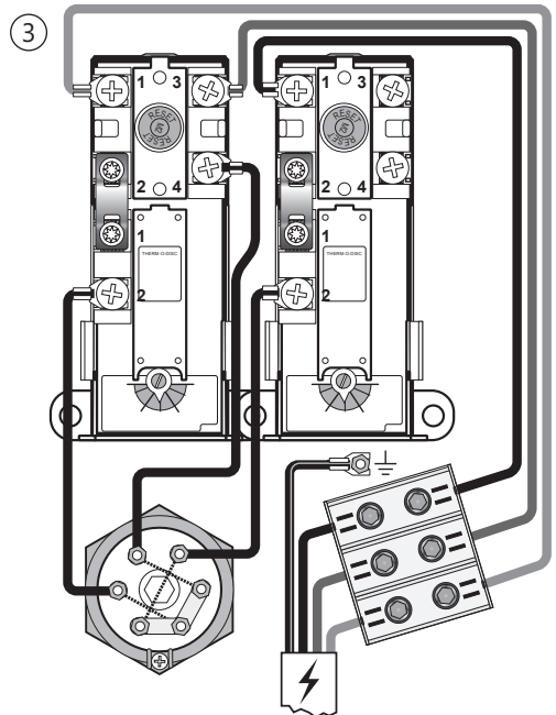
KytKentäkaavio - 9 kW - 3x400V Alasäiliön vaihtoeht. kytKentä - HUOM Nollajohdin EI OLE mahdollinen.
