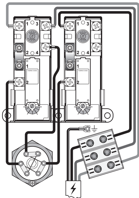
Kytkeäntärsiö - 9 kW - 3x230V Aläsäiliön normaalikytkentä
