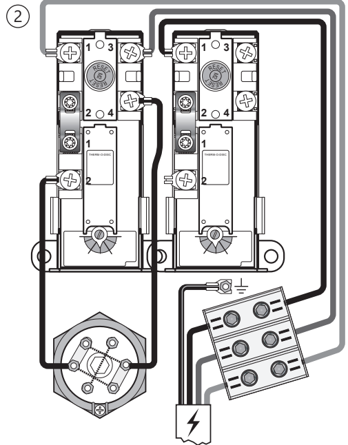
KytKentäkaavio - 6 kW - 3x230V Alasäiliön vaihtoehtoinen kytKentä
