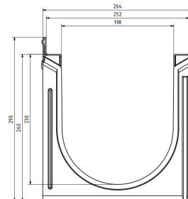
Poikkileikkaus, mitat mm
