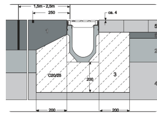
E600 Betonipeti C20/25 · 200 mm
