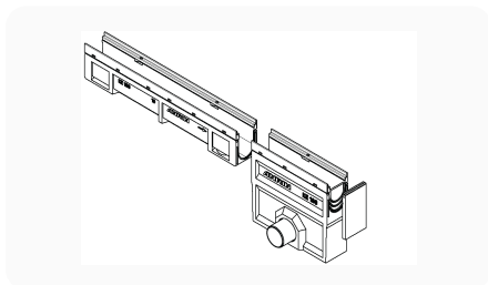
Hiekanerotin päädyssä
