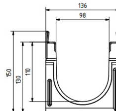
Poikkileikkaus, mitat mm
