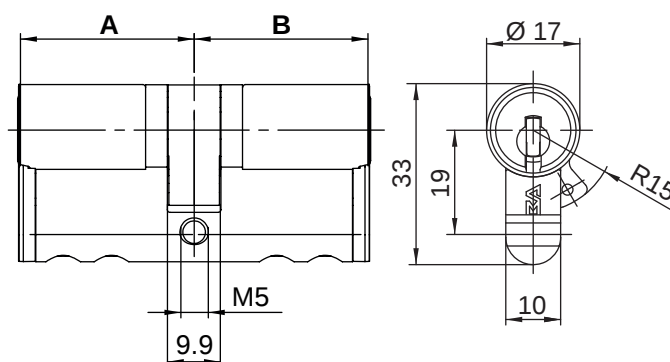
M1415 mit Frontabdeckung in Zylinder-Farbe
