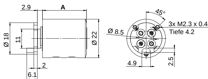
M1008C mit Ring Element in Zylinder-Farbe für Kaba 20
