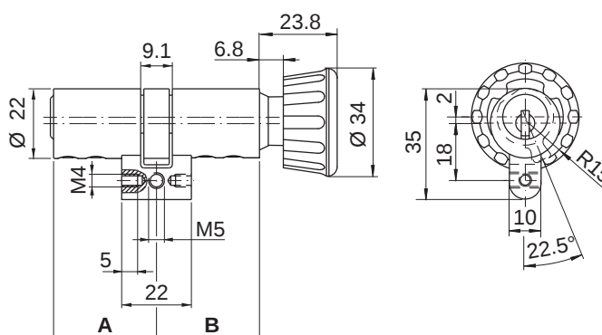
M1519 mit Drehknopf traditionell
