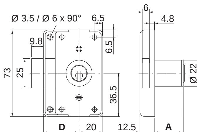
Bandung rechts / Schliessrichtung links
