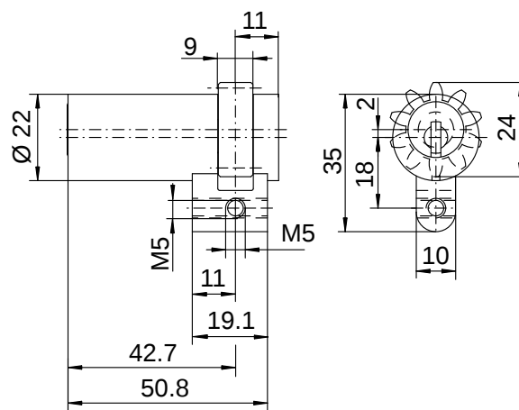
M1514DEP mit Ring Element in Zylinder-Farbe für Kaba 20
