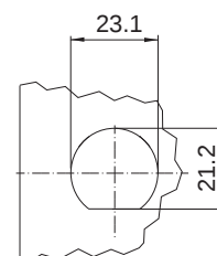
Zylinderausschnitt
