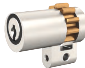
M1514 mit Ring Element schwarz + Multilock-Mitnehmer (ML)
