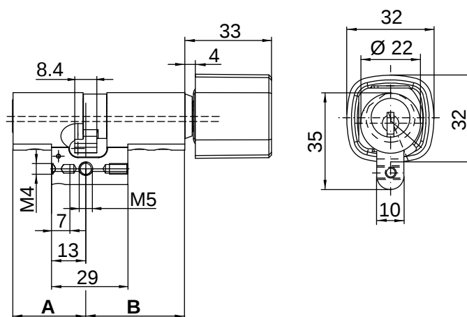
M1519A mit Design-Drehknopf + Ring Element schwarz
