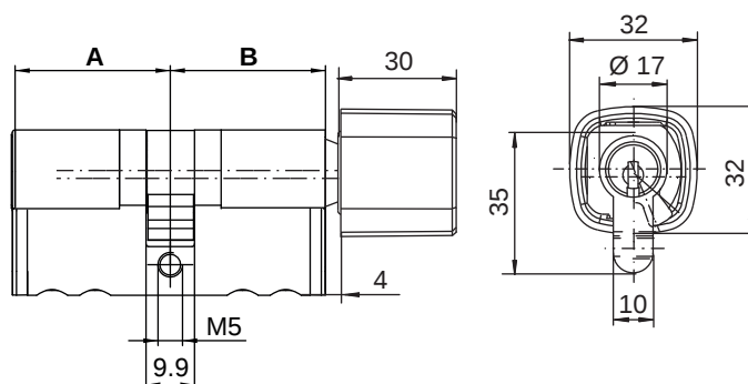
M1419 mit Design-Drehknopf
