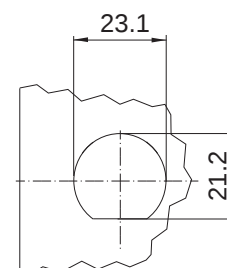
Zylinderausschnitt
