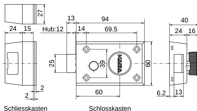
Bandung DIN rechts / Schliessrichtung links
