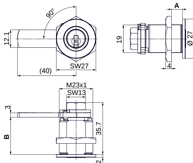
Bandung DIN rechts / Schliessrichtung links
