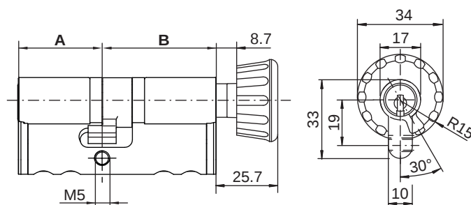
M1419 mit Drehknopf traditionell
