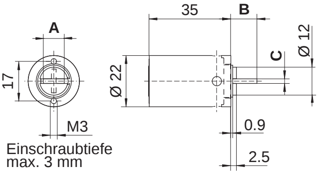
mit Ring Element in Zylinder-Farbe für Kaba 20
