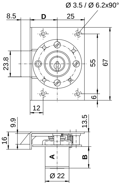
Bandung rechts / Schliessrichtung links
