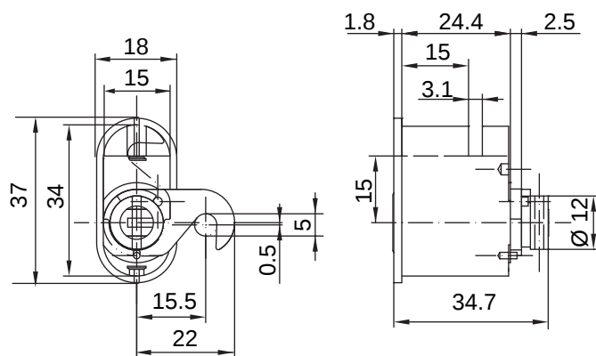
Bandung links / Schliessrichtung rechts
