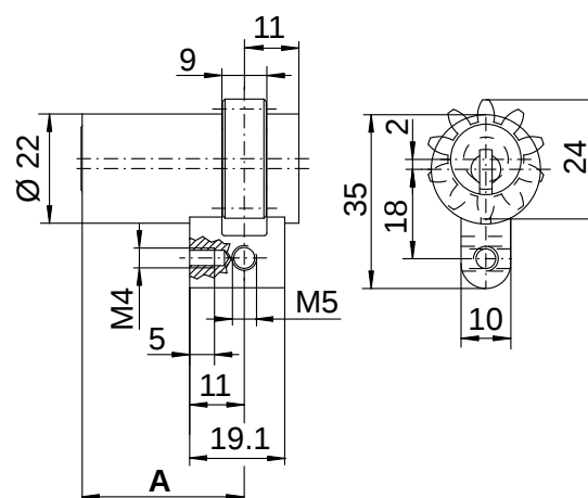
Multilock-Mitnehmer: Modul m = 2 Zähnezahl z1 = 10
