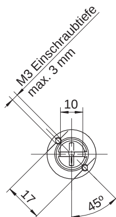
M1262G mit Ring Element in Zylinder-Farbe für Kaba 20
