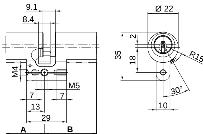
M1515A mit Ring Element in Zylinder-Farbe für Kaba 20
