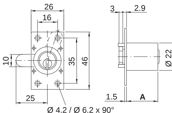
Bandung DIN rechts / Schliessrichtung links
