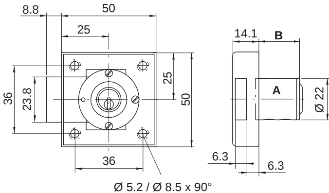
Riegel 0 mm verlängert - Bandung rechts / Schliessrichtung links
