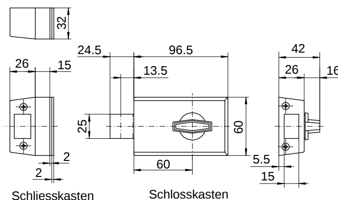
Schliesskasten
