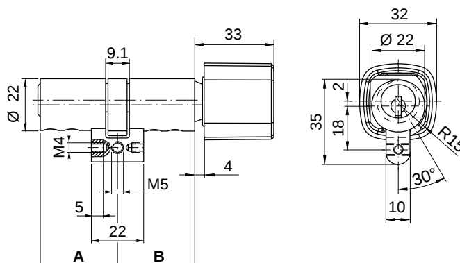
M1519P mit Design-Drehknopf + Ring Element schwarz
