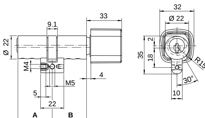
M1519 mit Drehknopf Design (DK)
