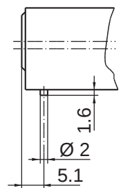
Kontaktstift
