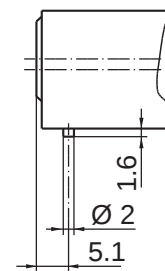
Kontaktstift
