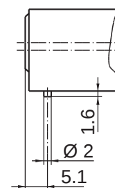
Kontaktstift
