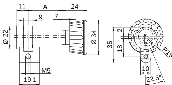
M1514D mit Drehknopf traditionell
