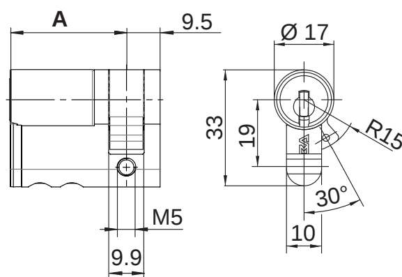
M1414 mit Frontabdeckung in Zylinder-Farbe
