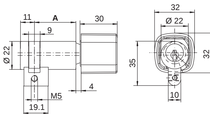
M1514D mit Design-Drehknopf
