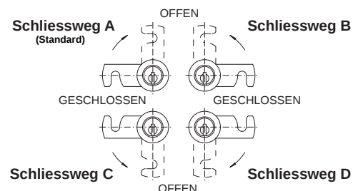
Bandung DIN rechts / Schliessrichtung links
