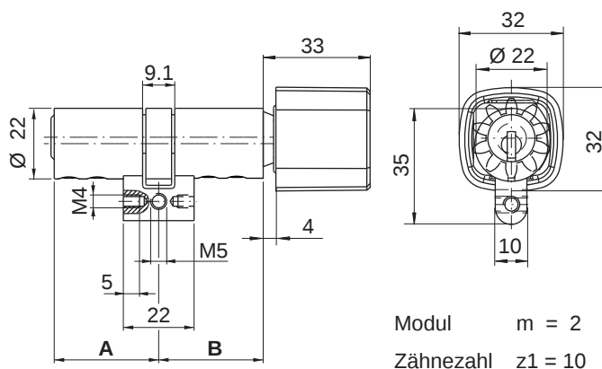
Drehknopf Design (DK) + Multilock-Mitnehmer 2214H-3 (MLCH)
