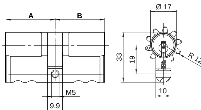
M1415 mit Bestelloption Multilock-Mitnehmer (ML)
