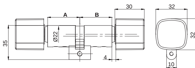
M1519D mit Design-Drehknopf
