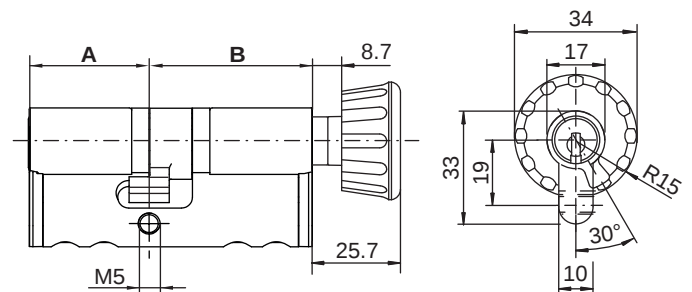
M1419A mit Drehknopf traditionell
