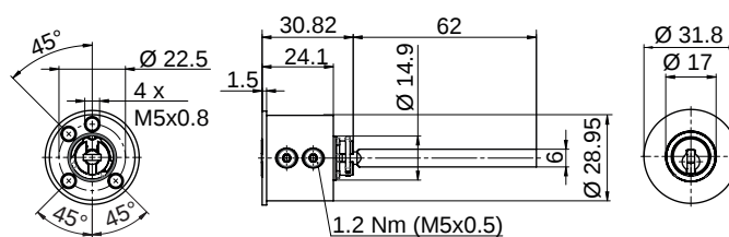
M1007 mit Ring Element in Zylinder-Farbe für Kaba 20
