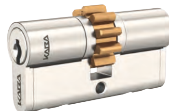
M1415 mit Bestelloption Multilock-Mitnehmer (ML)
