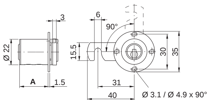
Bandung DIN rechts / Schliessrichtung links
