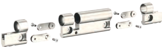
Zusammenbau Profilzylinder
