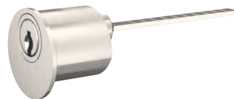
M1007B mit Ring Element in Zylinder-Farbe für Kaba 20
