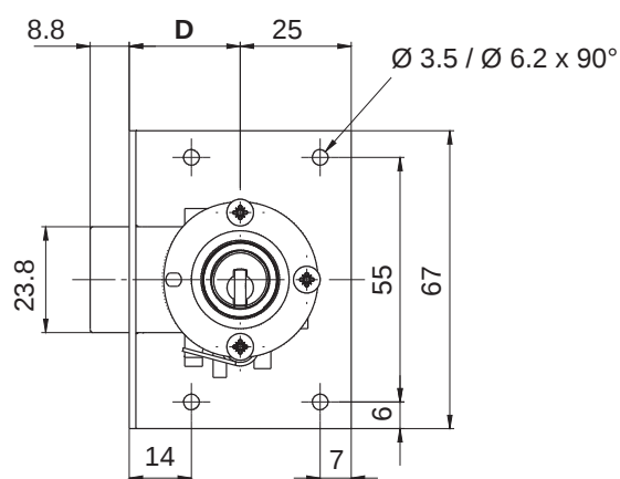
Bandung links / Schliessrichtung rechts
