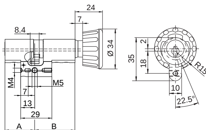
M1519A mit DK trad. + Ring Element in Zyl.-Farbe für Kaba 20
