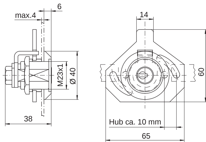
M2024 mit Ring Element in Zylinder-Farbe für Kaba 20
