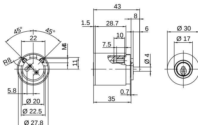
M1507 mit Ring Element in Zylinder-Farbe für Kaba 20
