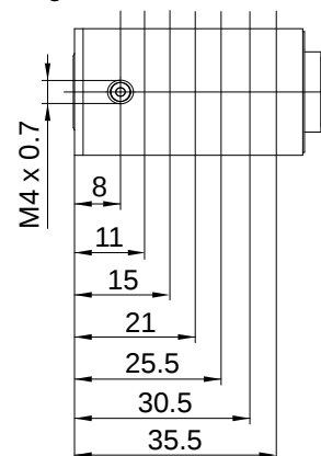
Bohrungen 1 2 3 4 5 6 7
