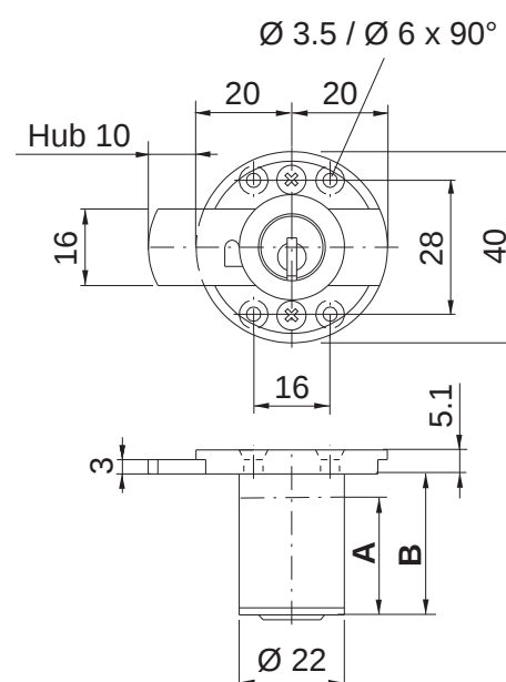
Bandung rechts / Schliessrichtung links
