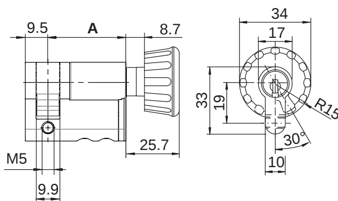
M1414D mit Drehknopf traditionell
