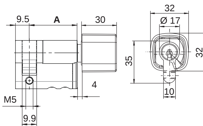
M1414D mit Design-Drehknopf
