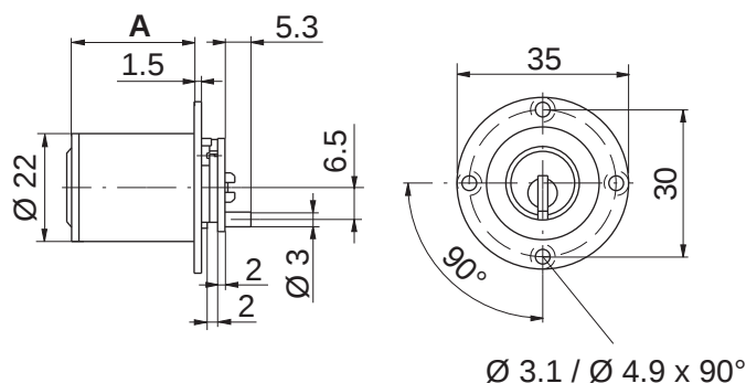
MXVI mit Ring Element in Zylinder-Farbe für Kaba 20
