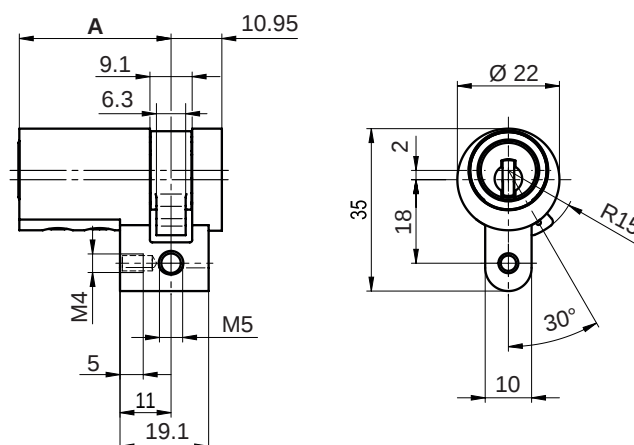
Mitnehmer schmal modular (N)
