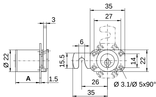
Bandung DIN rechts / Schliessrichtung links
