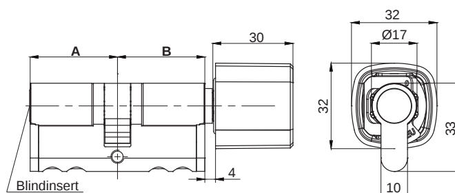
M1419P mit Design-Drehknopf
