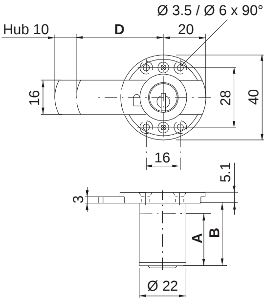
Bandung rechts / Schliessrichtung links
