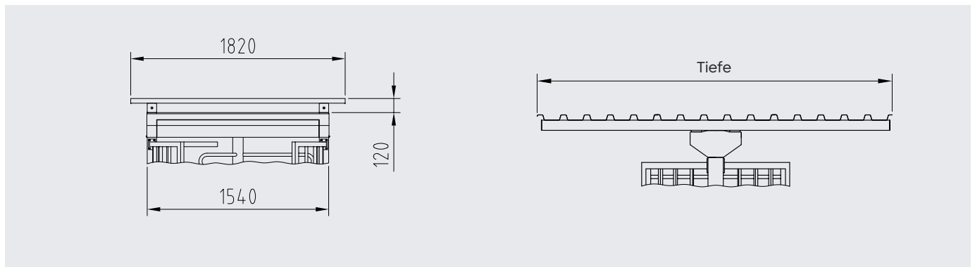
Dach D1 – mit Trapezblechabdeckung
