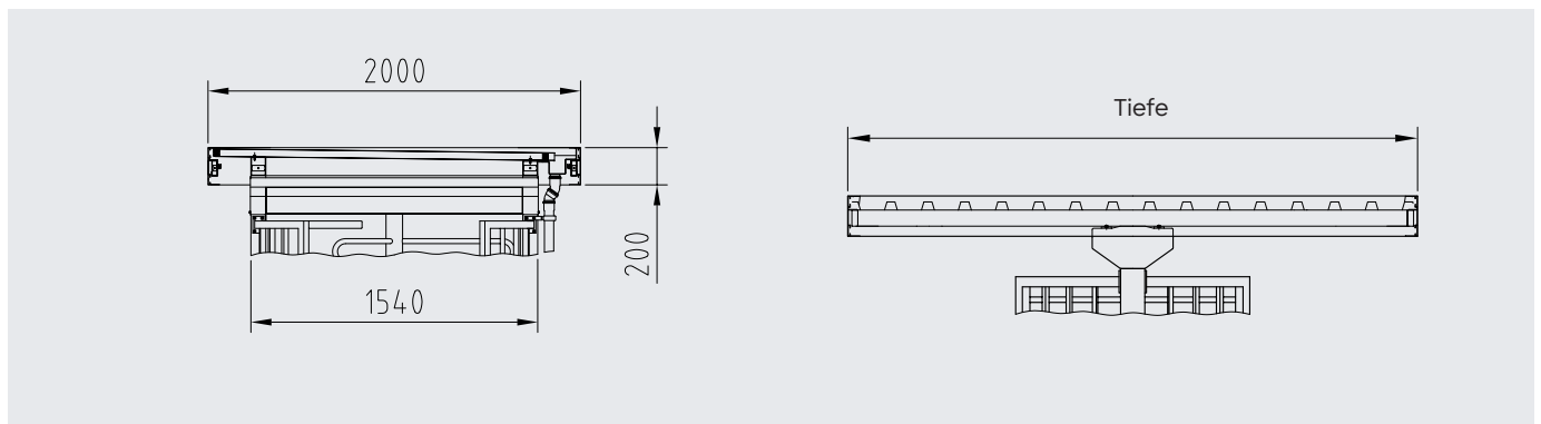
Dach D2 – mit Trapezblechabdeckung, Dachrandprofil und Wasserablauf
