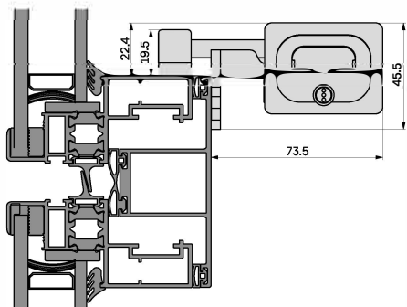
Etrier de supports pivotement INCLUS
