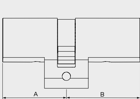
Doppelzylinder-Rundprofil 22 mm Steglänge immer fix 22 mm
