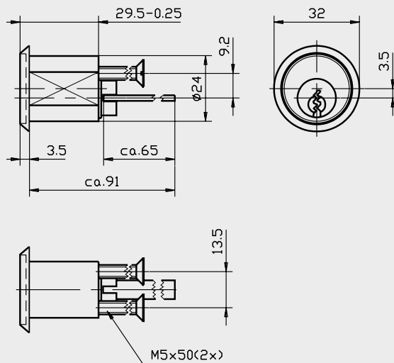
Außenzylinder AZ/AG208
