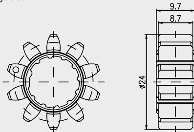
ZR10 Zahritzel mit 10 Zähnen
