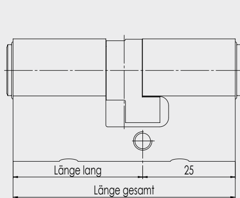
Doppel-Kurzzyylinder Europrofil 17 mm
