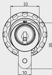
Längenkombinationen Drehknopfzylinder Kaba 8
