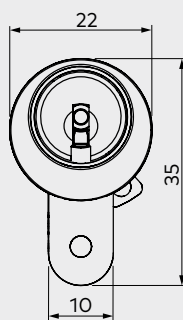
Längenkombinationen Doppelzylinder Kaba 8
