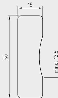
Ausschnitt Stahlzarge lt. ÖNORM B 5330-8 / Form B
