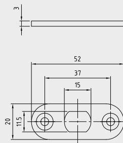
132/Stangenschließblech/DS
