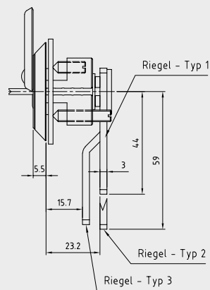
BMZ/5/SE/A1/PL inkl. Isolierung (PL) weiße Kunststoffabdeckung innen
