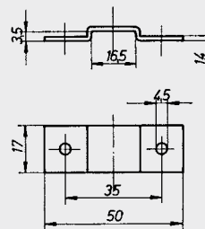
MZU/735/SCH
