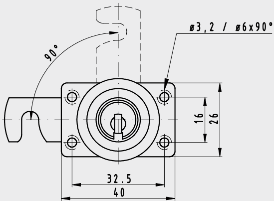
Anschraubplatte BS38 horizontal, rechts Verwendung für horizontal rechts und für vertikal links angeschlagen entspricht Schließweg A bzw. F
