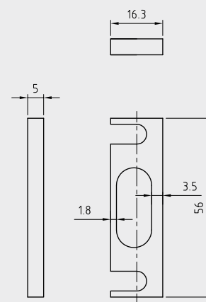
SB/Verstärkung/MV.Z/DS
