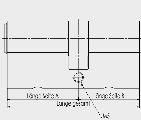
Doppelzylinder Europrofil 17 mm
