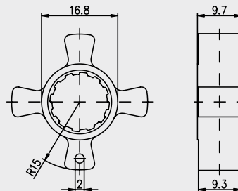
4-fach Mitnehmer
