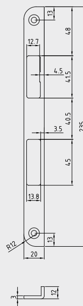
Winkelstulp
