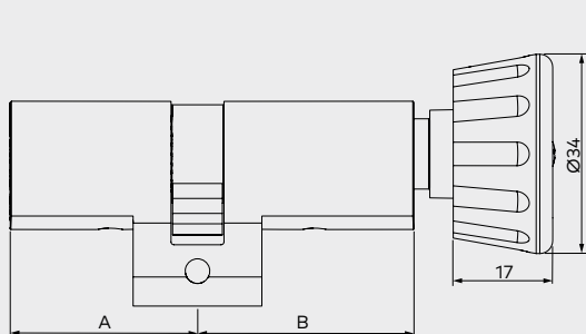
Drehknopfzylinder Rundprofil Steglänge immer fix 22 mm
