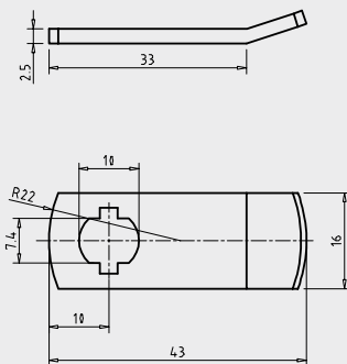
Zeichnungsnummer 210.201.780
