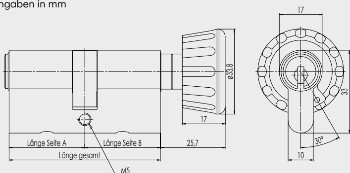
Drehknopfzylinder mit rundem Drehknopf (RK)
