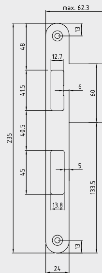
Lappenstulp
