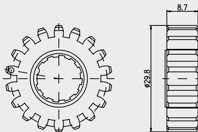
ZR18 Zahritzel mit 18 Zähnen
