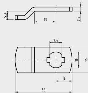
Zeichnungsnummer 210.201.781
