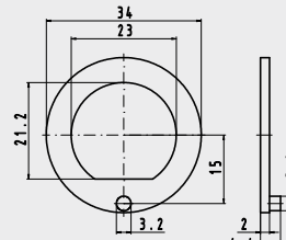
1031-24A
