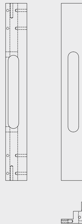
Frässhablone für SB/VAR.7
