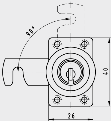
Anschraubplatte BS37 vertikal, rechts Verwendung für vertikal rechts und für horizontal links angeschlagen entspricht Schließweg B bzw. E
