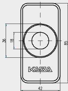
ROS/NO/E17/Ni/H
