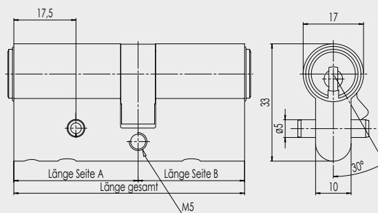
Doppelzylinder mit Ziehschutz
