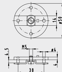
Vorrichtung für Stangenverschluss 3465
