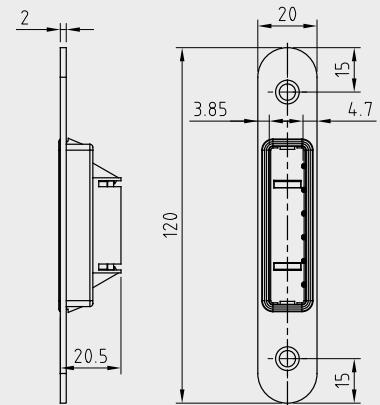
SB6
