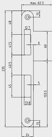
Lappenstulp
