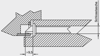
Einwandfreie Funktion nur bei Mindesteingriff lt. Zeichnung
