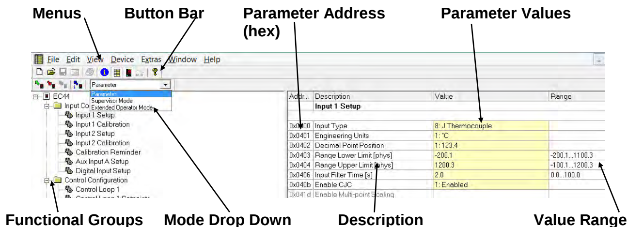
Figure 64. Main Parameter Screen
