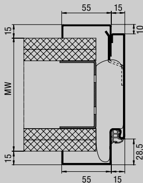
Profil 31103 s polodrážkou
