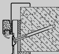
Diagonální upevnění S přídatnou zárubní Vario B53 jako 2-dílnou obvodovou zárubní (pórobeton)
