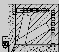
Rohová zárubeň Montáž do zdiva Hmoždinkové ukotvení do zdiva
