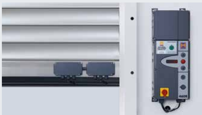
Bezdrátová přenosová jednotka // NOVINKA Volitelná výbava pro přenos signálů z pláště vrat na řídicí jednotku přes Bluetooth – místo šroubovicového vedení. Napájení zajišťuje výkonná baterie. Pro řídicí jednotky: 445 R / 460 R
