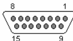
Identificación pineado conector DB15
