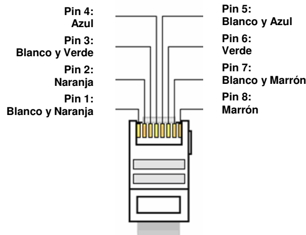
Pineado conectores RJ45
