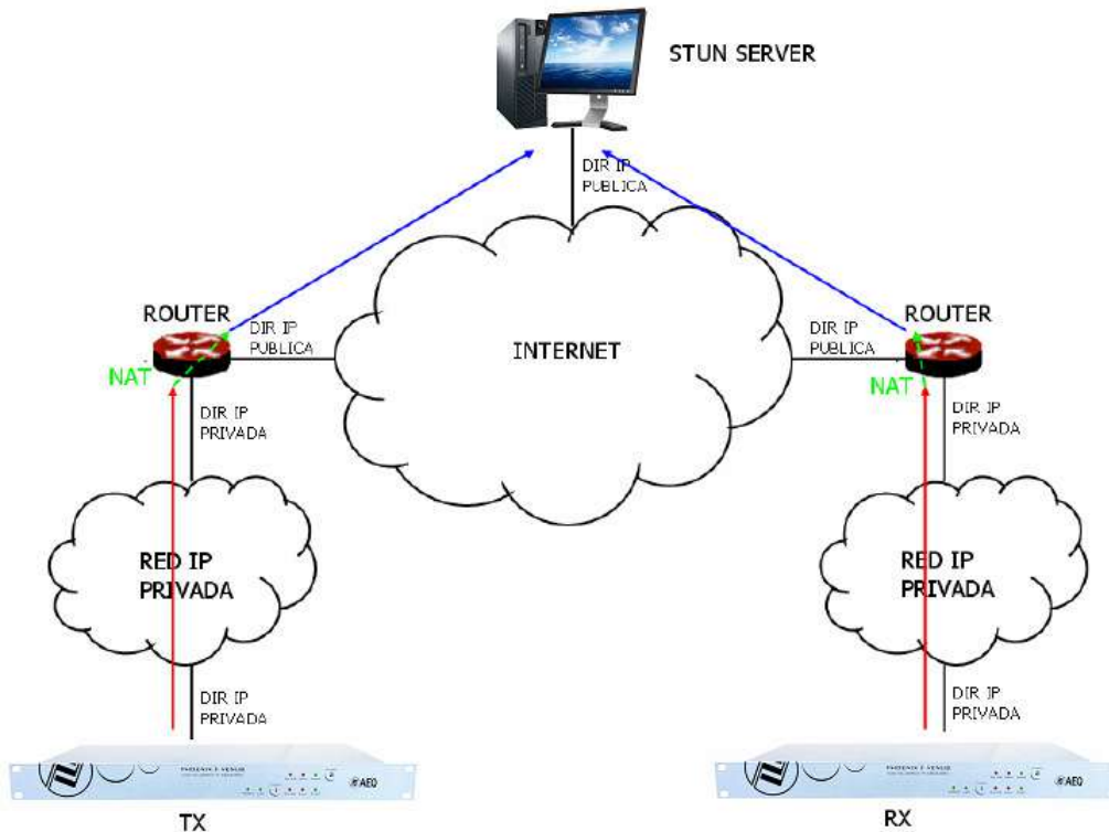
Registro en servidor STUN
