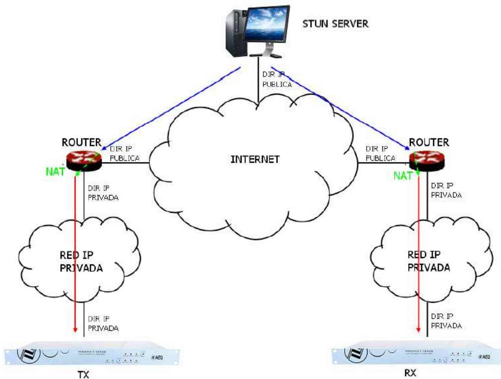
Notificación del servidor de los correspondientes NAT detectados
