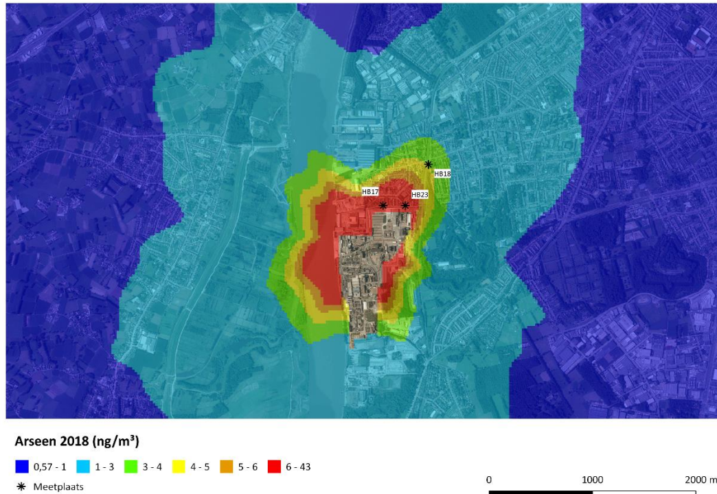
Figuur 2: Modellerings As-concentratie in Hoboken, op basis van meetresultaten 2018, uitgevoerd door VMM
