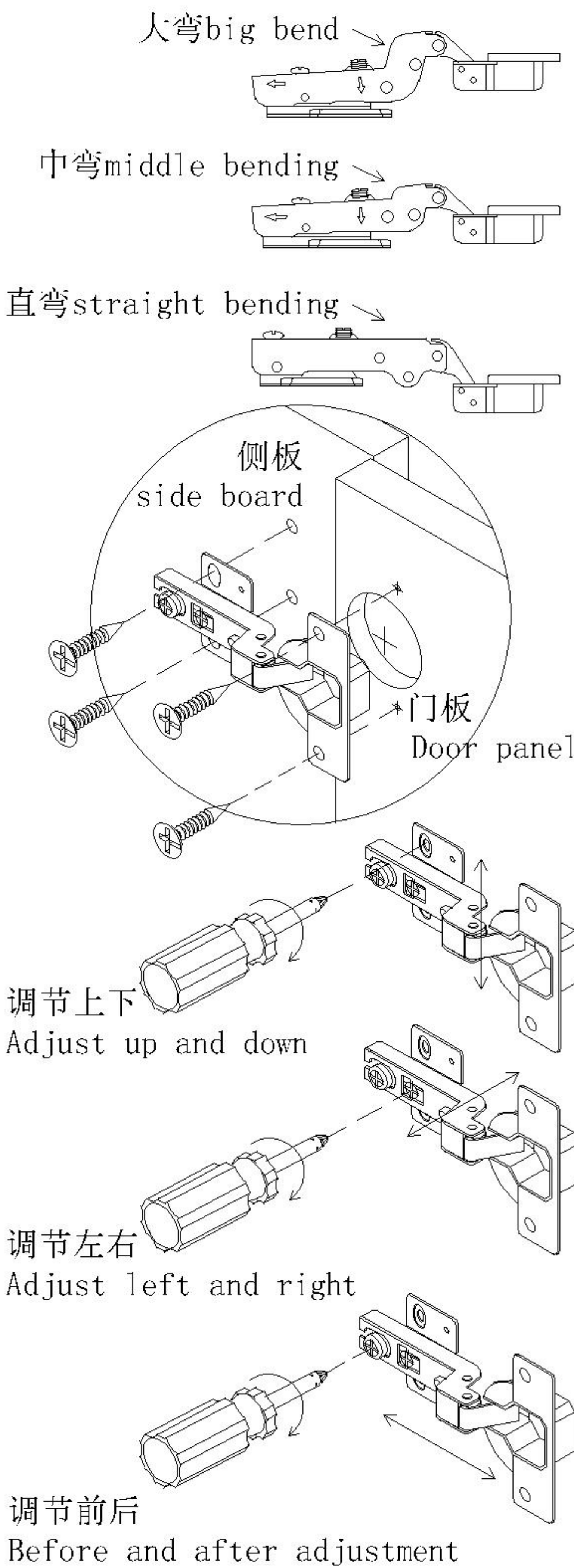
门铰 Hinge
