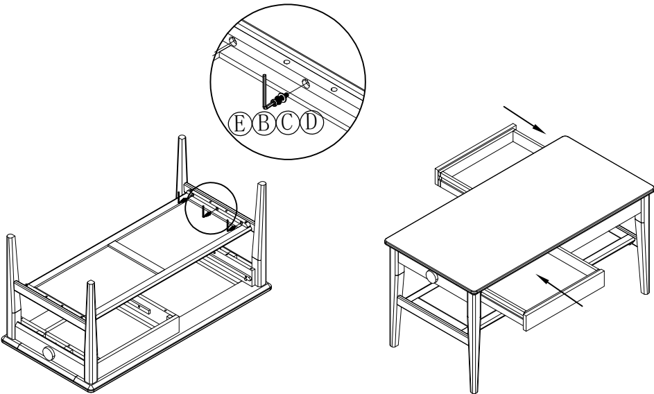
第二步：隔板与腿框连接
