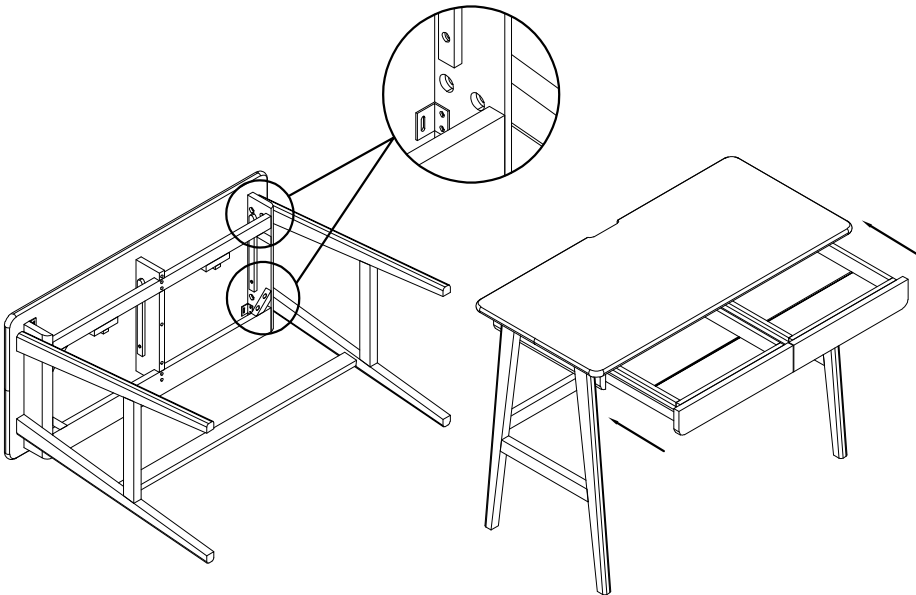
第二步：桌框与腿框组装
