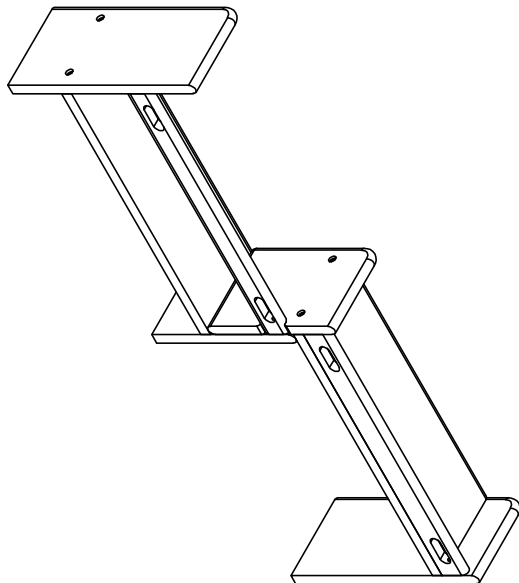
禾沐小书架（伸缩组合） 组装图
