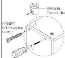
塑料螺母 Plastic Nut
