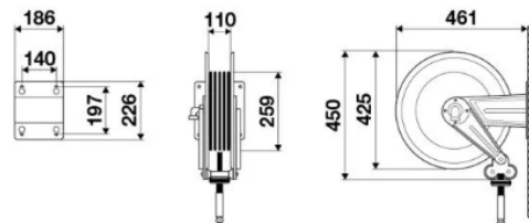
DIMENSÕES CARRETÉL EM ABS (mm)
