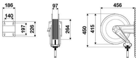
DIMENSÕES CARRETÉL EM AÇO (mm)
