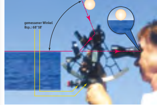
In nach Stellung der Alhidade, die mit der Hand verschoben wird, wird ein größerer oder kleinerer Winkel gemessen.
