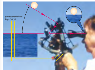
Sonnenstehung im Spiegelbild des Sextanten.
