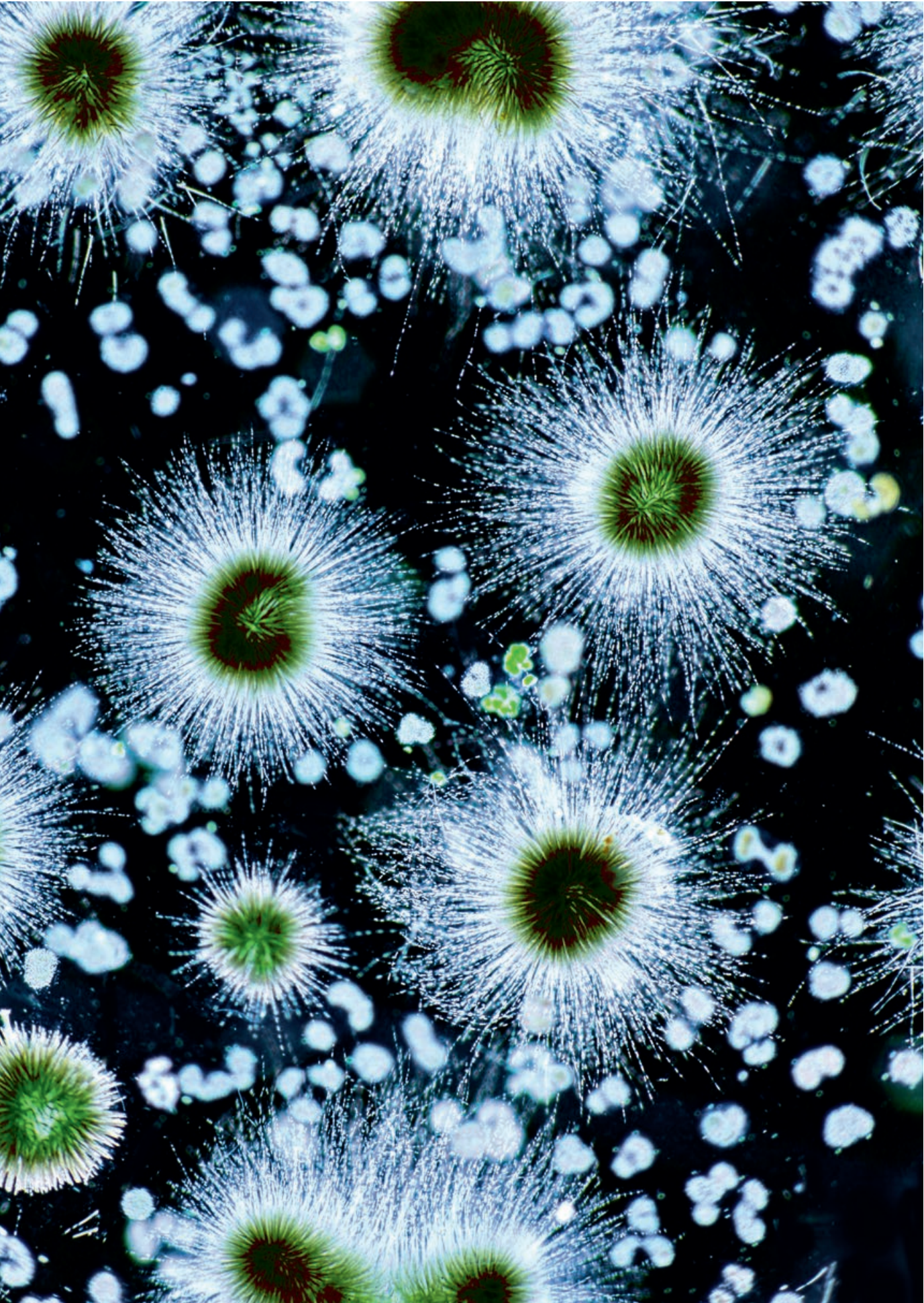
Gloeotrichia-Cyanobakterien haben die besondere Fähigkeit, durch Gasblasen an der Oberfläche von Seen zu treiben.
