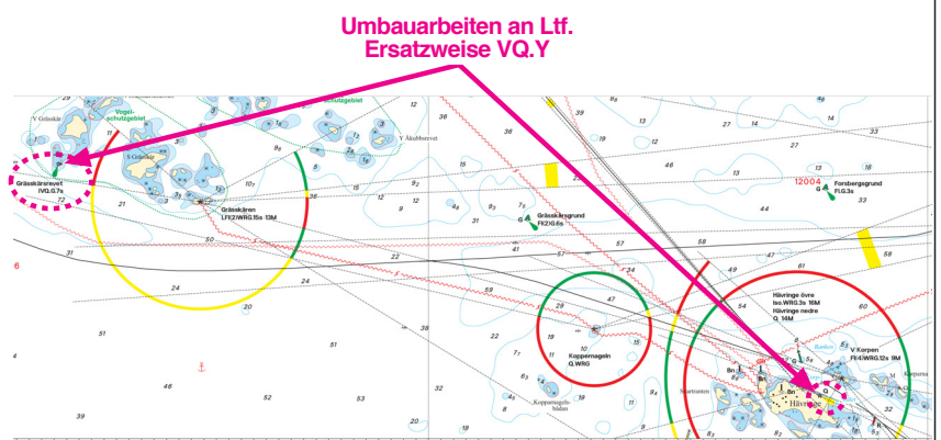
Abbildung 7 - Satz 12 Ausschnitt aus Karte 08 Umbau von Leuchtfuern - Ersatzbefeuerung
