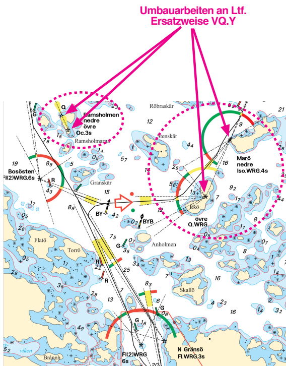
Abbildung 6 - Satz 12 Ausschnitt aus Karte 03 Umbau von Leuchtfuern - Ersatzbef.
