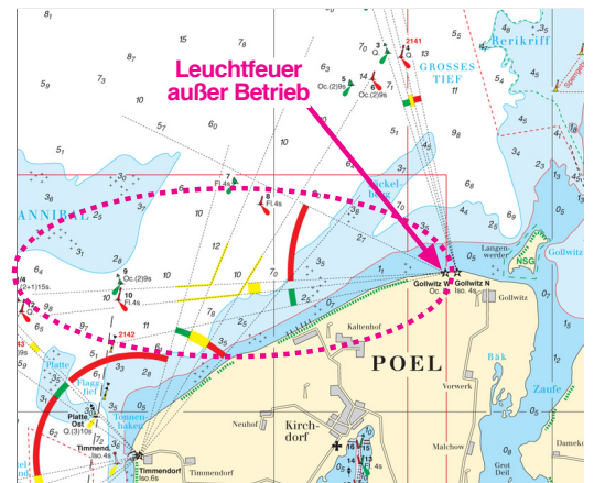
Abbildung 4 - Satz 2 Ausschnitt aus Karte 04 Lf. Gollwitz-W außer Betrieb
