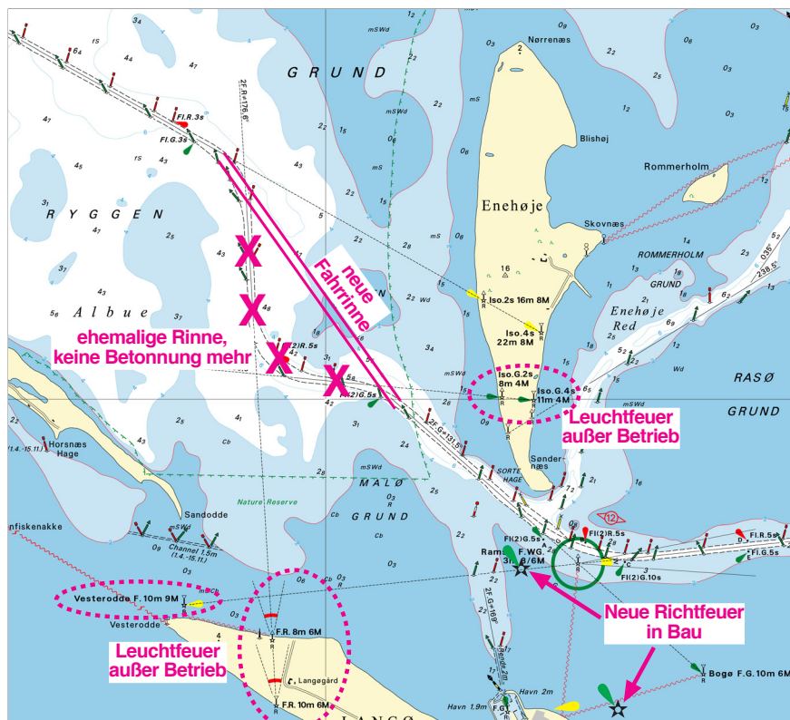
Abbildung 3 - Satz 1 + Satz 4 Ausschnitt aus Karte 23 Neuer Fahrwasserabschnitt nach Nakskov
