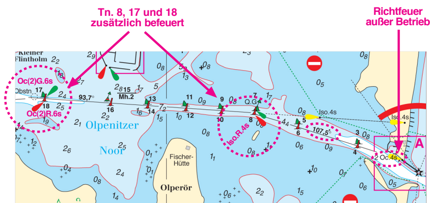
Abbildung 1 - Satz 1 Ausschnitt aus Karte Schlei 1 Rchtf. Schleimünde außer Betrieb, Tonnen befeuert
