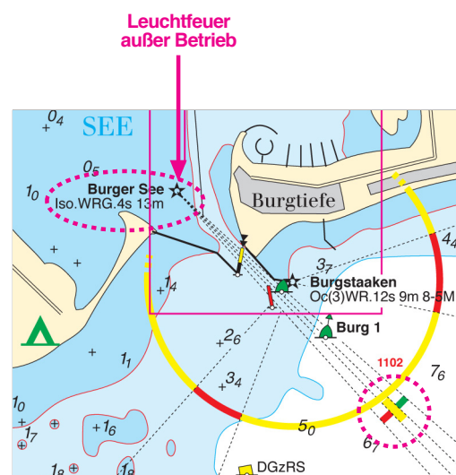
Abbildung 2 - Satz 1 + Satz 2 Ausschnitt aus Karte 07A / 01A Ltf. Burger See außer Betrieb
